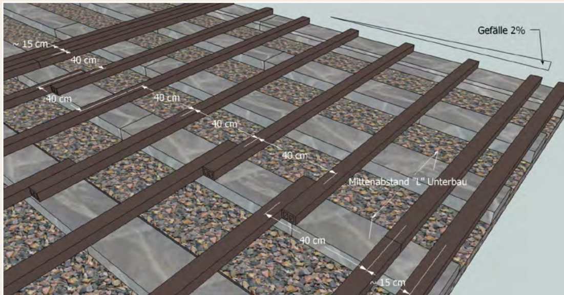
Bild 1: Unterbau und Unterkonstruktion / Verlängerung der UK
